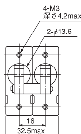
2極Hハンドル
