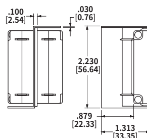
LEGターミナルバリア (Z)
