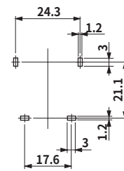
P板取付穴参考寸法図
