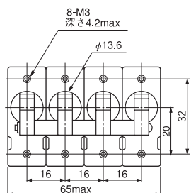
4極Hハンドル
