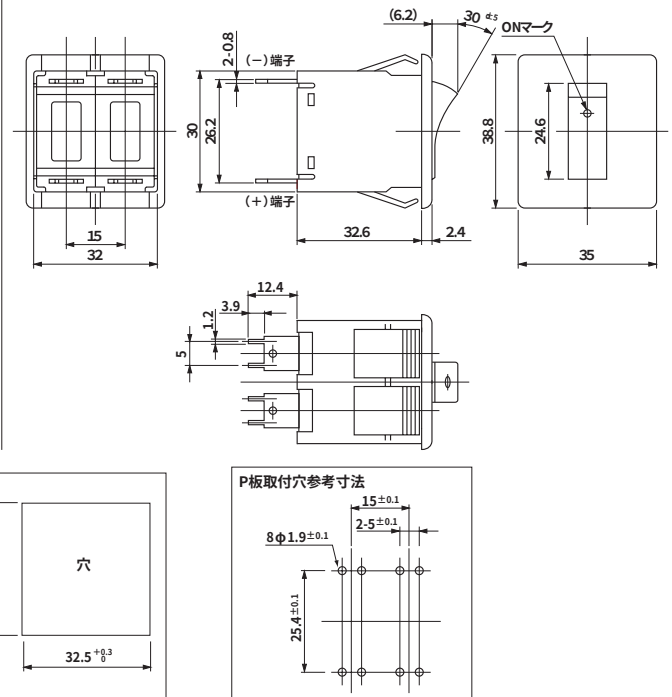
パネル取付参考寸法
