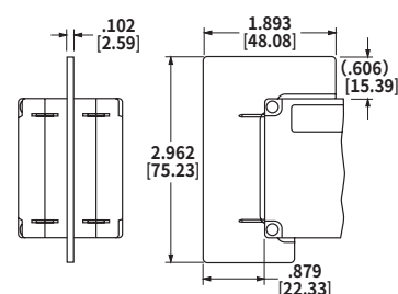
LEGターミナルバリア LEG 2極品にはターミナルバリアが付きません。
