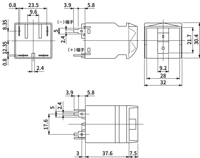
P板取付穴参考寸法図
