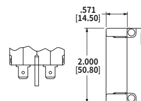
CEGターミナルバリア (B)
