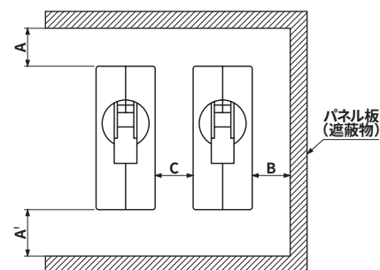
アーーククリアランス推奨値
