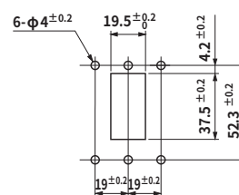
単ハンドル穴あけ寸法図
