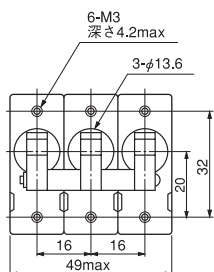
3極Hハンドル
