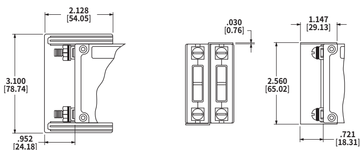
LELターミナルバリア (B)
