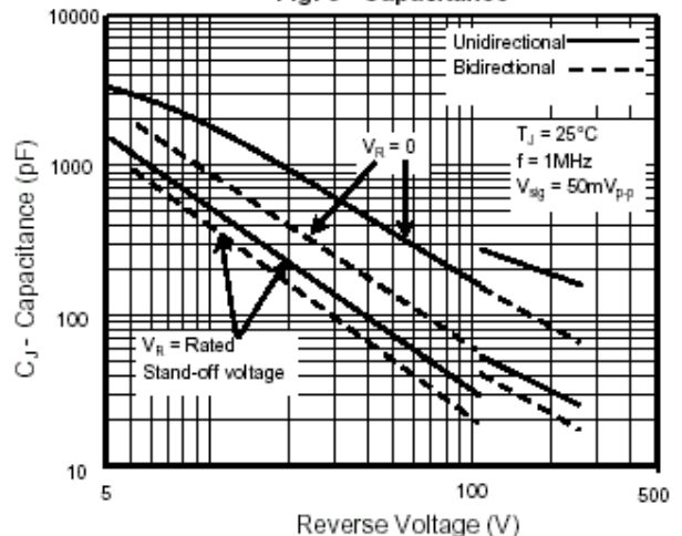
Fig. 6 - Capacitance
