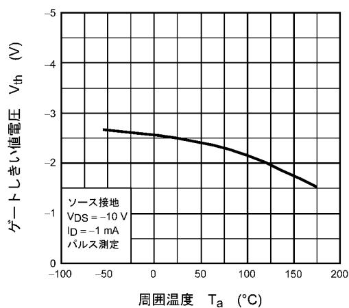
図 8.9 V_{th} - T_a (注8)
