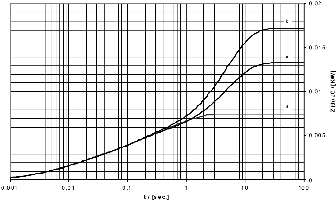
Transienter innerer Wärmewiderstand für DC/ Transient thermal impedance Z_{thJC} = f(t) for DC
