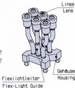
Einbaubeispiel für 1304.1002 Mounting Example for 1304.1002
