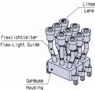
Einbaubeispiel für 1304.1001 Mounting Example for 1304.1001
