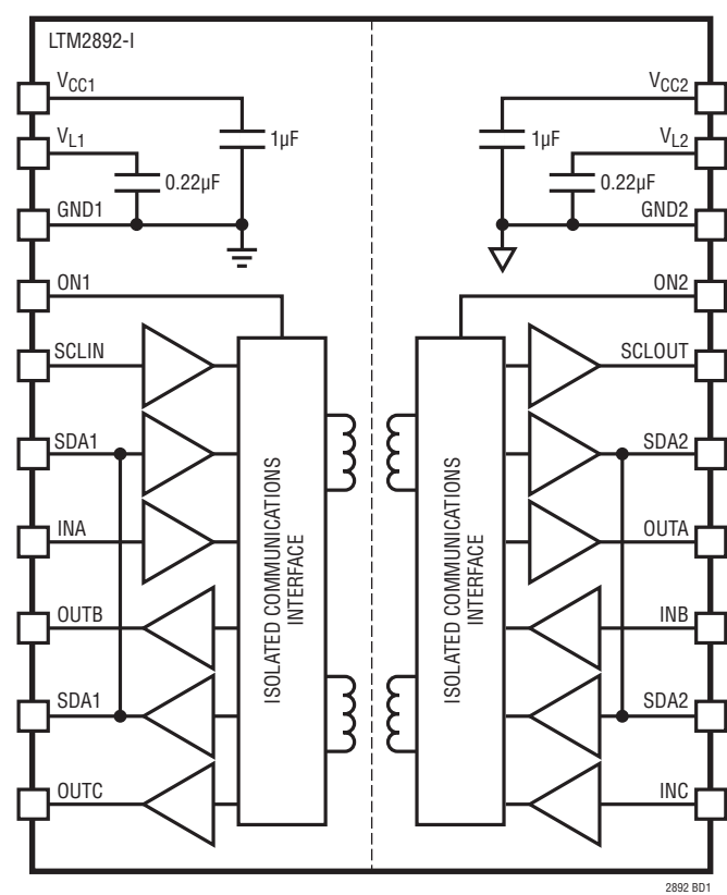
LTM2892-I
