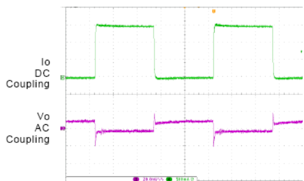
12. Load Transient
