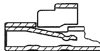
断面 "A"- "A" (SECT) (175152-4)
