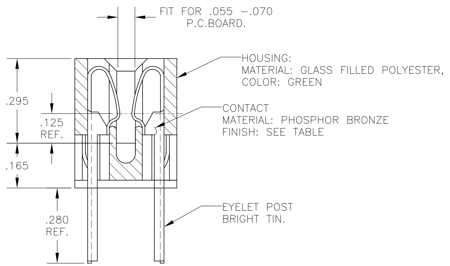
SECT A-A
