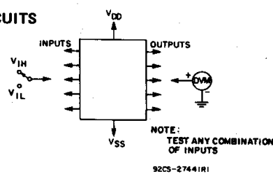
Fig. 10 - Input voltage.
