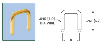
.040 (1.0) PINS
