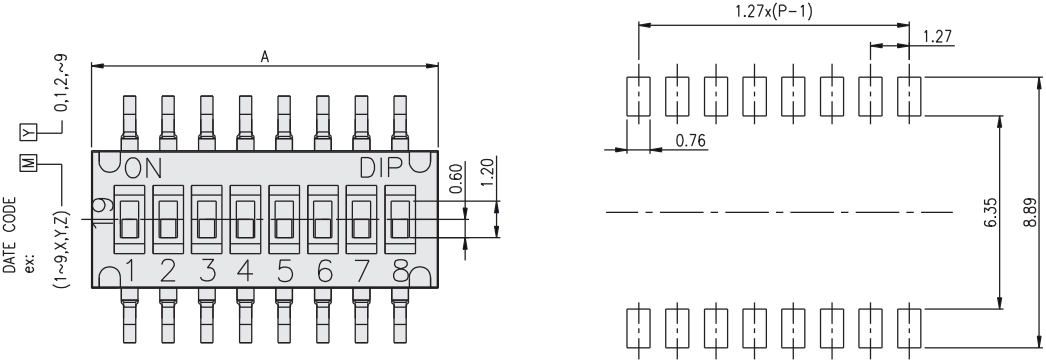
P.C.B. LAYOUT
