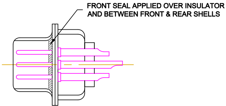
DETAIL A-A
