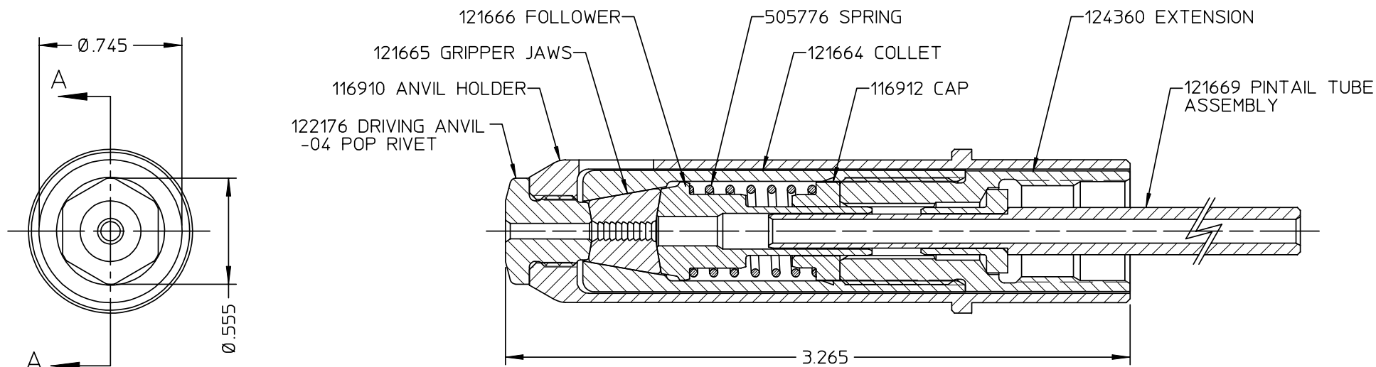
SECTION A-A
