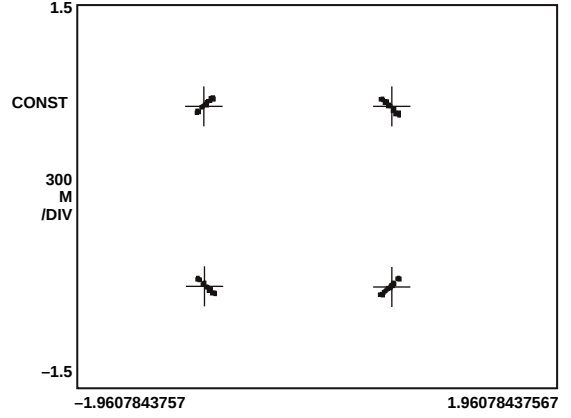
TRACE A: CH 1 MSK1 MEAS TIME
