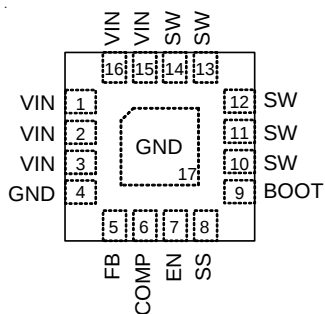
WQFN-16L 3x3
