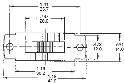
DP3T
