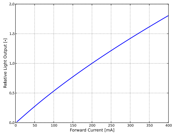
LUXEON CoB: LHC1 – xxxx – 1202
