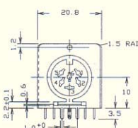
D6 6 Pin 240° right angle PCB mounting DIN socket.
