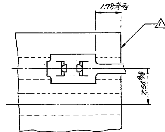
矢視「B-B」 (ケーブル端での圧着一例である。)
