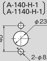
パネル穴明け寸法 Panel drilling dimensions
