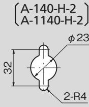
パネル穴明け寸法 Panel drilling dimensions
