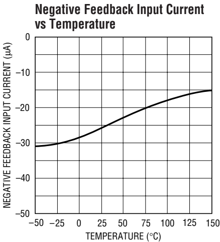
LT1513 • G06
