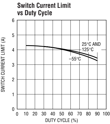
LT1513 • G02
