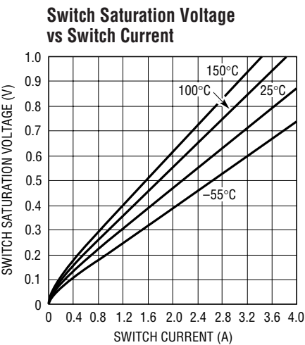
LT1513 • G01
