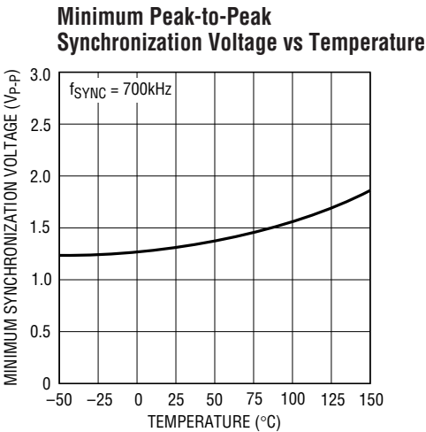
LT1513 • G04
