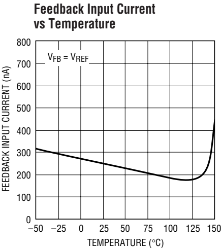
LT1513 • G05
