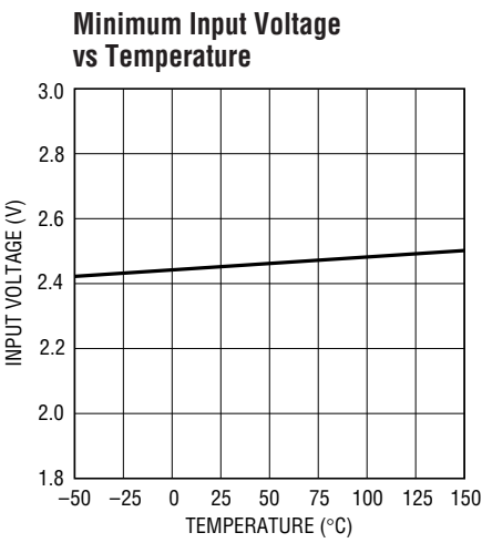
LT1513 • G03
