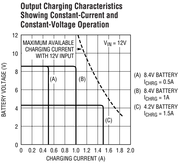
1513 G07
