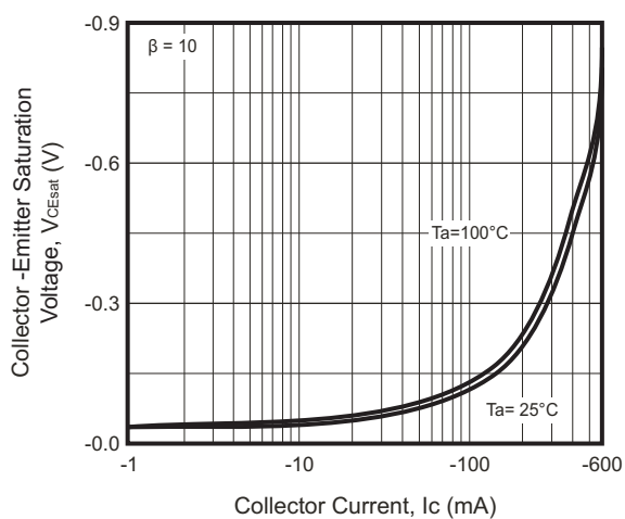
Fig.3 - V_{CEsat} - I_c
