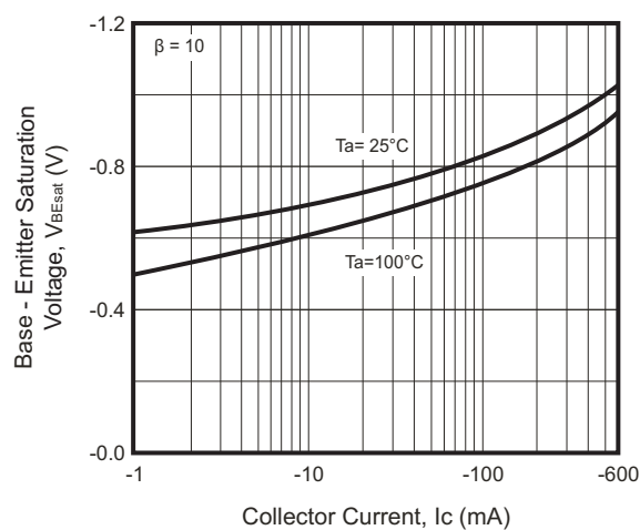
Fig.4 - V_{BEsat} - I_c
