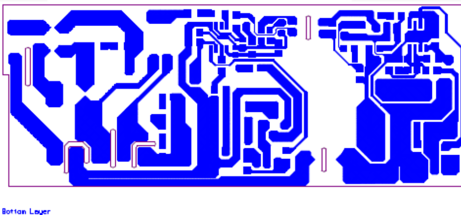
Figure 27. Bottom Layer
