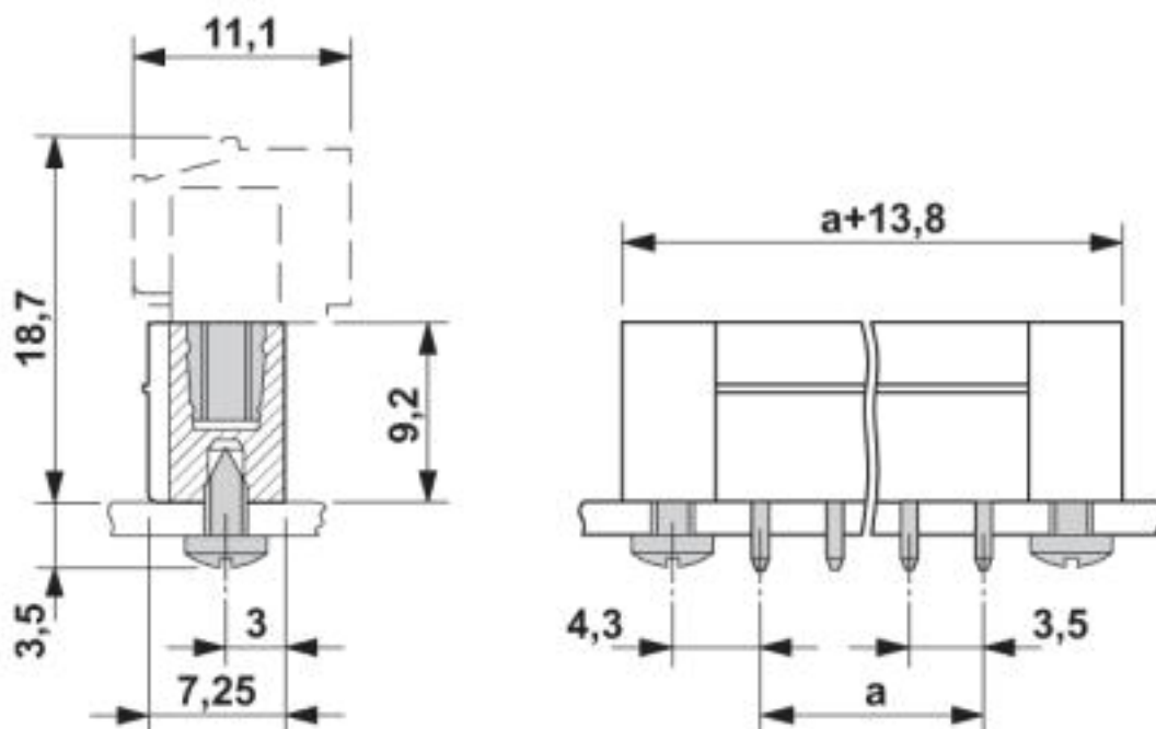
Maßzeichnung
