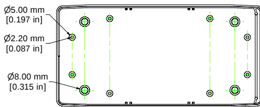
LID - INSIDE
