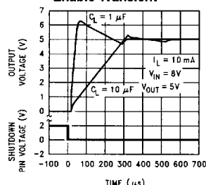
LP2951 Enable Transient
