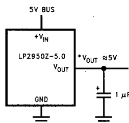
5 Volt Current Limiter
