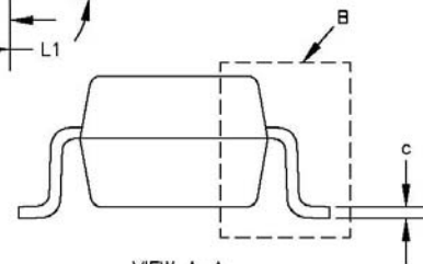
VIEW A-A
