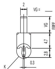
K DETAIL 2:1
