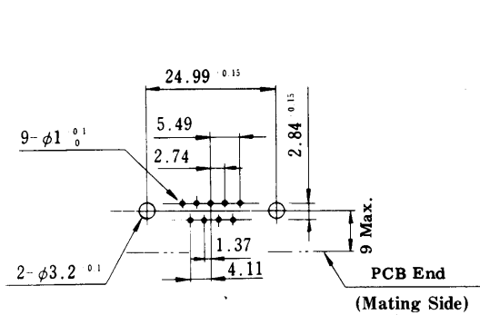
RDDE-9
