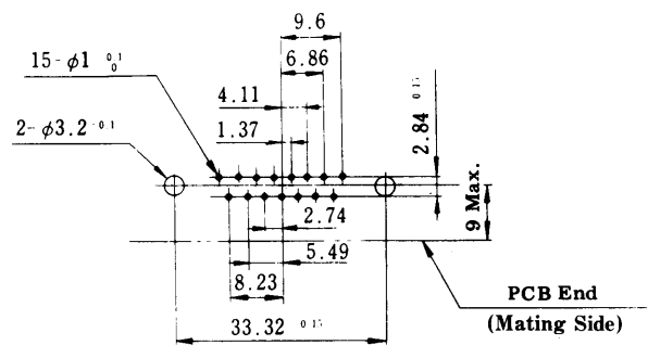
RDAD-15
