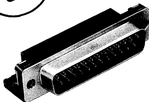
CL211-5170-8-05 RDBD-25PE1/M2.6(05)
