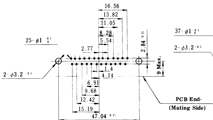
RDBD-25
