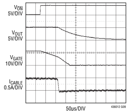
Entering Sleep Mode (LTC4360-1)
