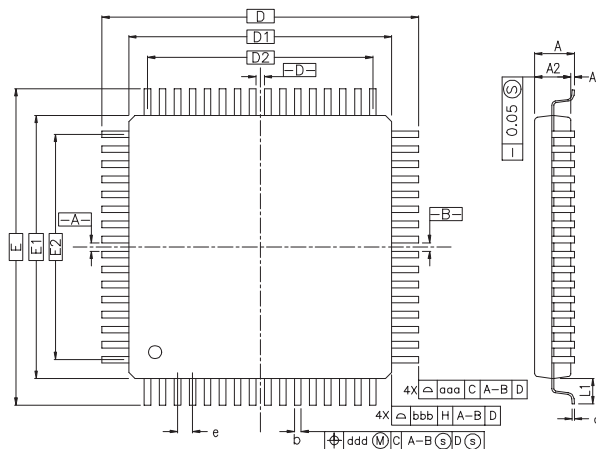
SYMBOL MILLIMETER INCH MIN. NOM. MAX. MIN. NOM. MAX. A — — 1.60 — — 0.06 A1 0.05 — 0.15 0.002 — 0.005 A2 1.35 1.40 1.45 0.053 0.055 0.057 D 16.00 BSC. 0.630 BSC. D1 14.00 BSC. 0.551 BSC. E 16.00 BSC. 0.630 BSC. E1 14.00 BSC. 0.551 BSC. R2 0.08 — 0.20 0.003 — 0.008 R1 0.08 — — 0.003 — — θ 0° 3.5° 7° 0° 3.5° 7° θ1 0° — — 0° — — θ2 11° 12° 13° 11° 12° 13° θ3 11° 12° 13° 11° 12° 13° c 0.09 — 0.20 0.004 — 0.008 L 0.45 0.60 0.75 0.018 0.024 0.030 L1 — 1.00 REF — 0.039 REF S 0.20 — — 0.008 — —
