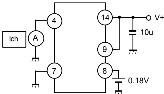
Test Circuit 5 Ich
