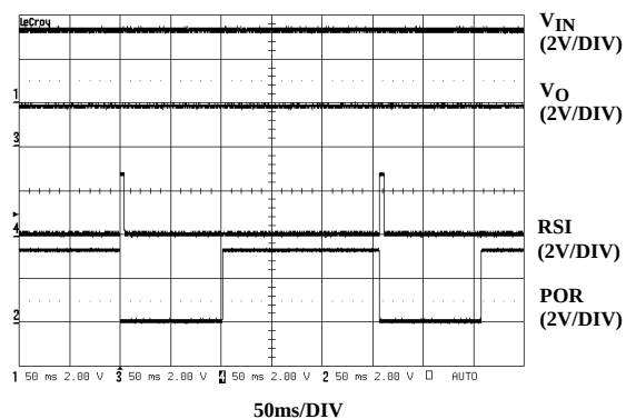
FIGURE 7. POR FUNCTION
