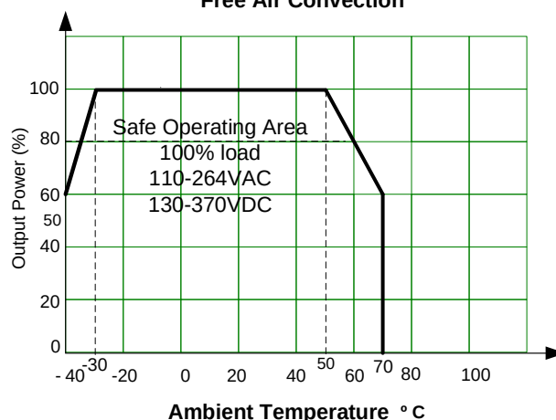
AME60-12SMJZ & AME60-15SMJZ Free Air Convection
