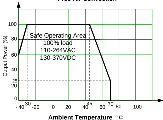
AME60-5SMJZ & AME60-5SMJZ Free Air Convection
