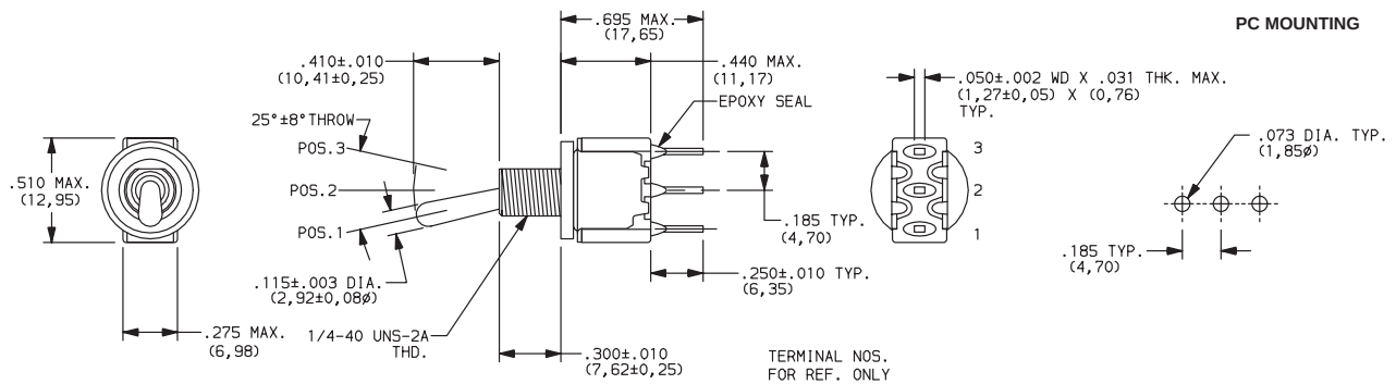
SPDT
