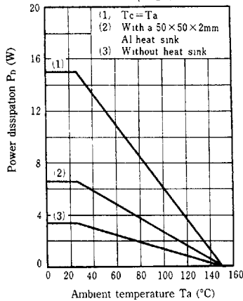
P_D - T_a (PU4117, PU4417)
