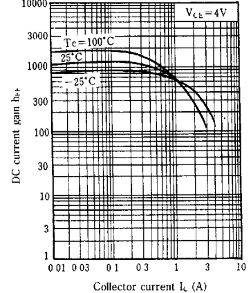
h_{FE} - I_C
