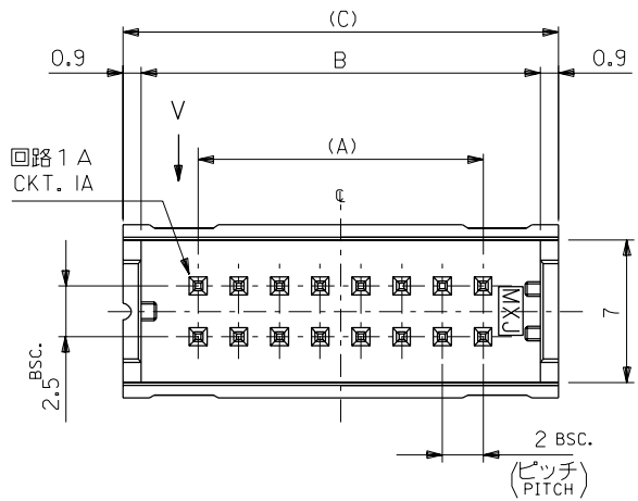
回路 1 A 表示 CKT. 1A IDENTIFICATION
