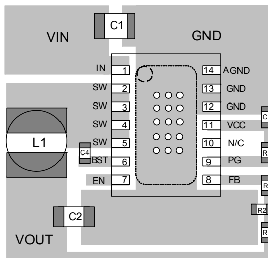
Top Layer
