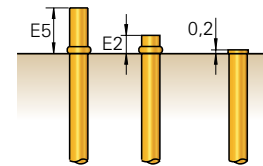
Einsatzbeispiel für KS-112 mit unterschiedlicher Kragenhöhe
