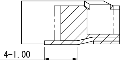
SECTION A-A(S=15/1)
