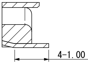
SECTION B-B(S=15/1)
