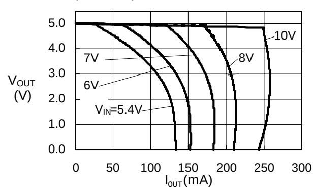
S-817B50A(Ta=25°C)
