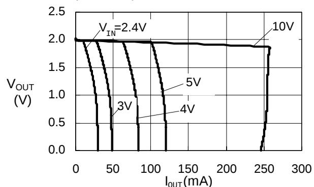
S-817B20A(Ta=25°C)
