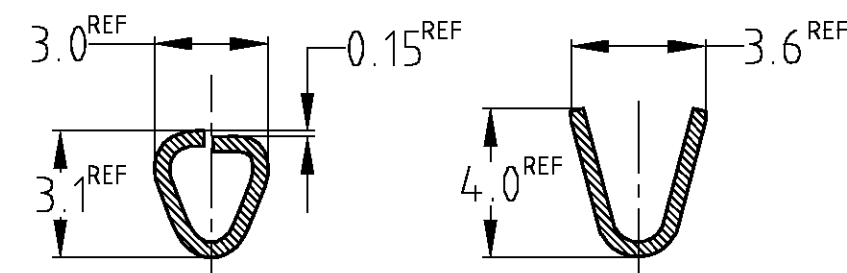
断面 B-B
