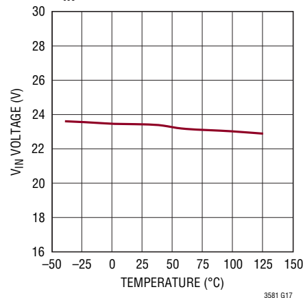
V_{IN} OVLO
