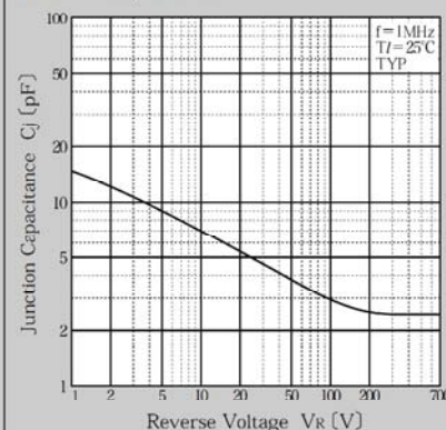
接合容量
