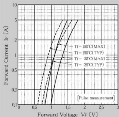
順方向特性
