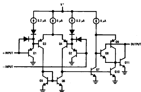
TL/H/5226-1
