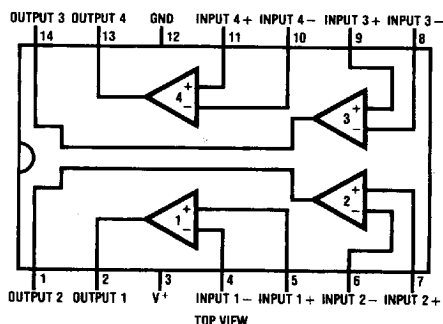
TL/H/5226-2
