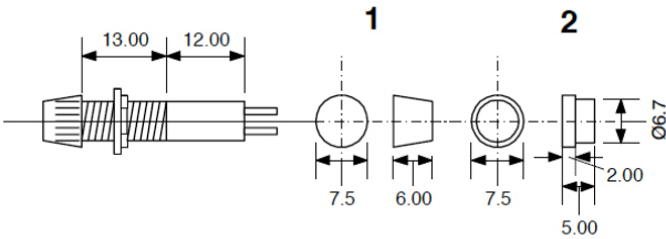
Body Dimensions
