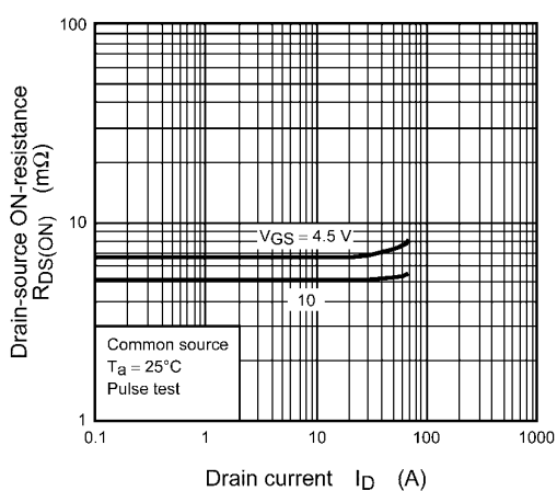
Fig. 8.5 R_{DS(ON)} - I_D
