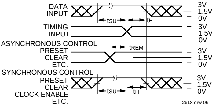
2618 drw 06
