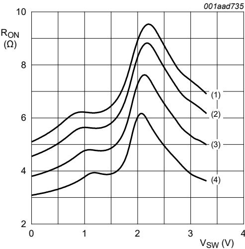
c. V_{CC} = 3.3\text{ V} ; I_{SW} = 64\text{ mA} ; V_{SW} = 0\text{ V}
