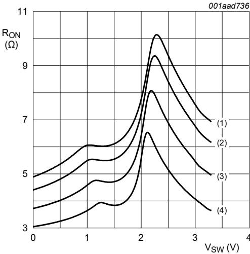
b. V_{CC} = 3.3\text{ V} ; I_{SW} = 24\text{ mA} ; V_{SW} = 0\text{ V}
